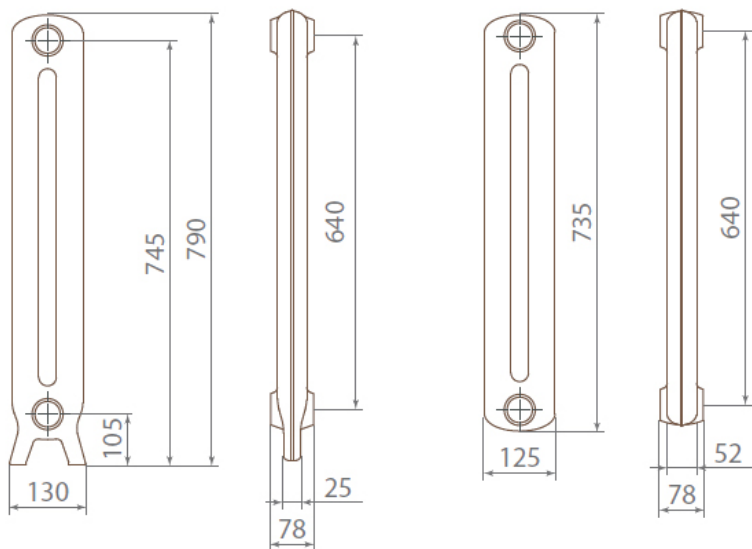
Чертеж секций радиатора EXEMET PRINCE 790/640
