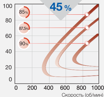
Эффективность DC-электродвигателя
