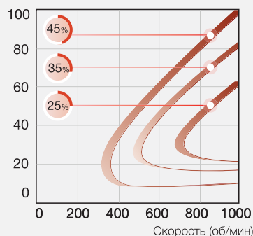
Эффективность AC-электродвигателя
