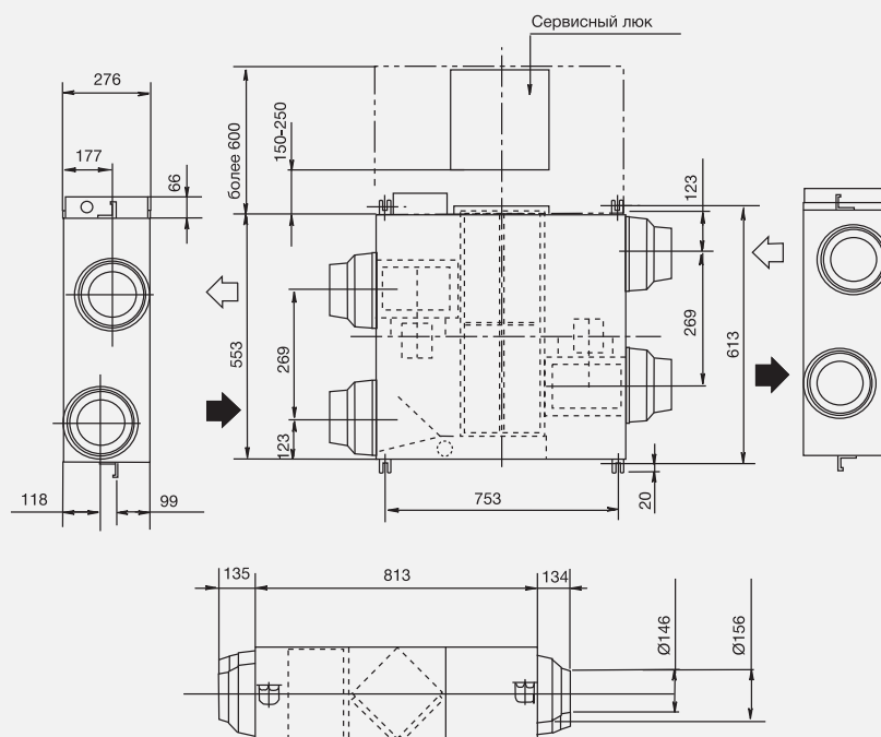
ERV0150AAN, ERV0260AAN
