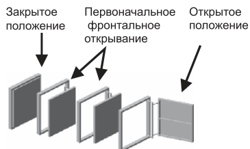
Схема открывания моделей «АТР», «ЕТР»
