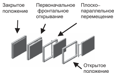
Схема открывания моделей «ЕСКР»
