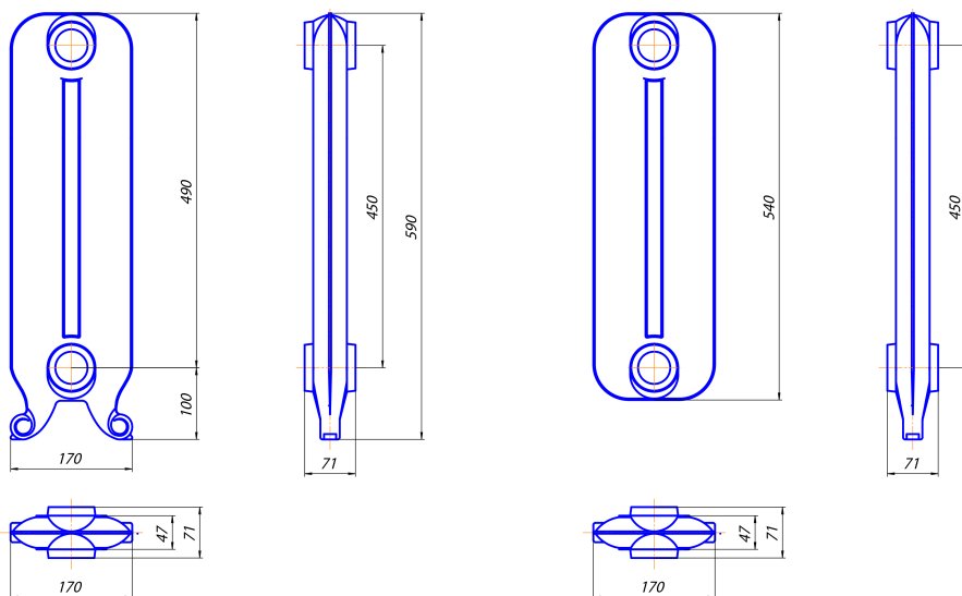
Чертеж секций радиатора EXEMET Queen 590/450
