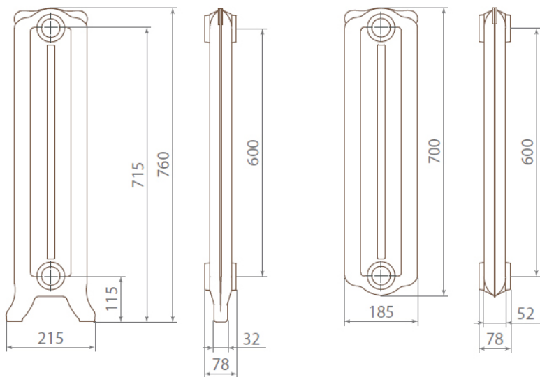
Чертеж секций радиатора EXEMET ROMANTICA 760/600
