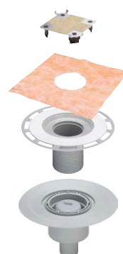
Вставка под плитку 4932.2 + надставной элемент 4925 + вертикальный трап 4926.5
