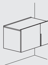
Mobile 90 maniglia verticale senza lavabo Filo 90 cabinet with vertical handle no washbasin cm 90 x 55 x 45 h pag. 22
