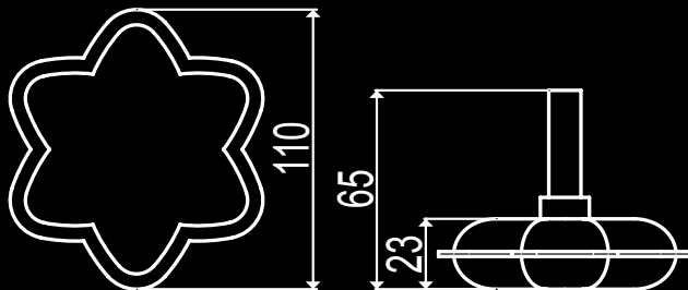
Appendino Fiore Fiore Hanger
