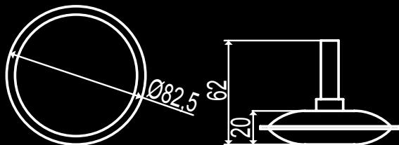
Appendino Tondo 82 Tondo 82 Hanger Ø: 82,5 mm - P: 62 mm
